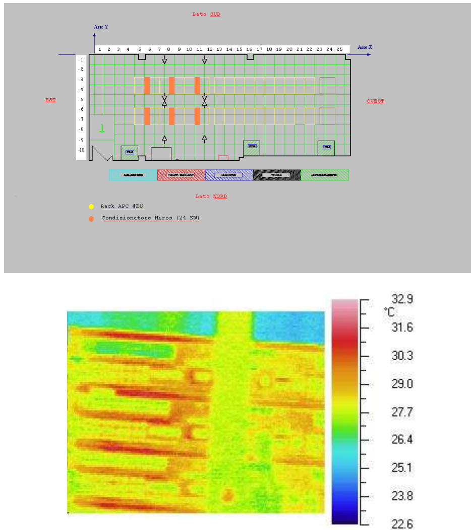
Fig. 9 – Studio di analisi termica della sala calcolo.
