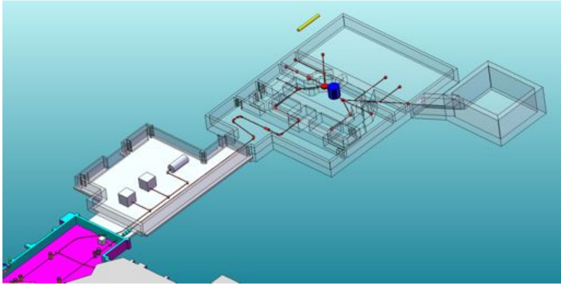
Fig. 3.22: Isometrico laboratorio Ciclotrone e layout di trasferimento e selezione del fascio esotico.
