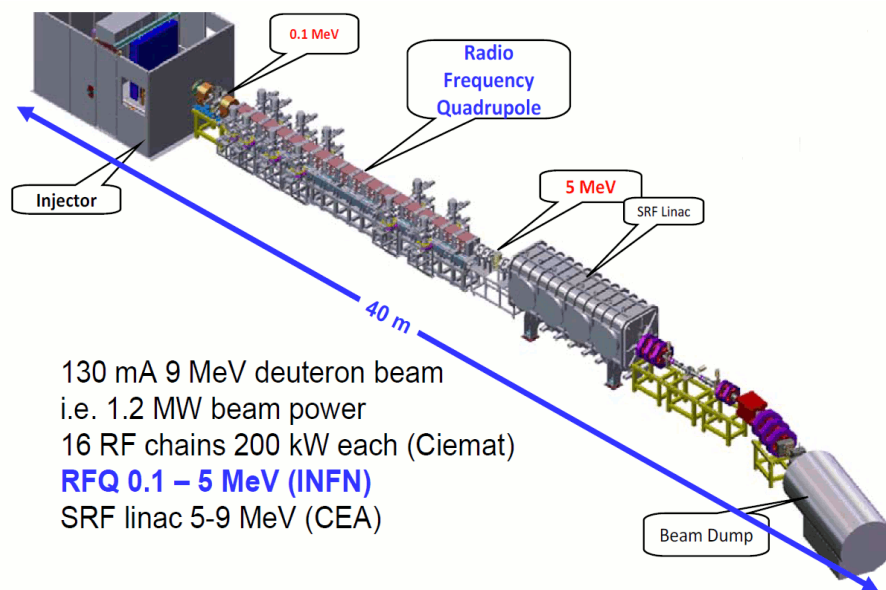
Fig. 3.18: Schema di IFMIF-EVEDA, il prototipo di acceleratore di deutoni ad altissima intensità per lo studio dei materiali per la produzione di energia da fusione nucleare.
