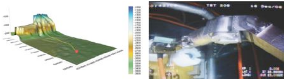
Fig. 4.29: Schema di posizionamento del cavo sottomarino nel sito di Capo Passero.
