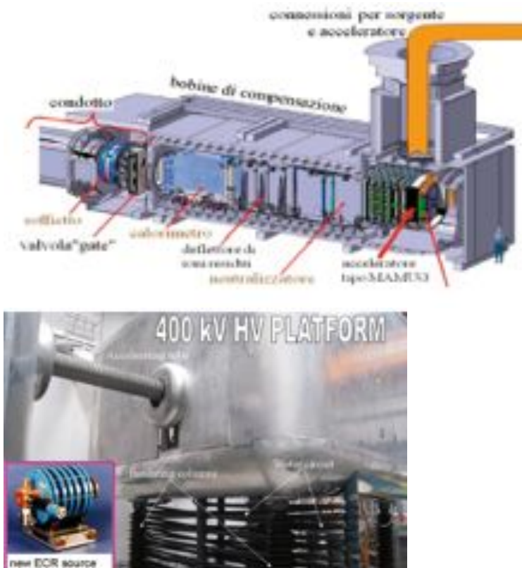
Fig. 4.16: La nuova sorgente ECR.
